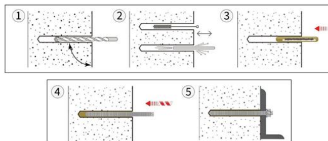
1-rasm. Kimyoviy ampulali anker o'rnatish jarayoni.
